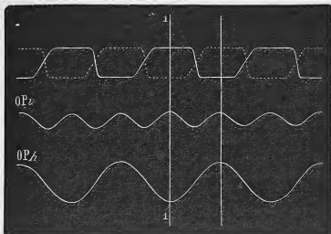
Fig. 22. — Les courbes supérieures, l'une pleine, l'autre ponctuée, représentent les phases d'appui et de lever des pieds droit et gauche. En lisant la figure de gauche à droite, chaque ascension d'une courbe indique le début d'un appui; la partie horizontale supérieure correspond à la durée de l'appui et la descente au lever du pied. Enfin la partie horizontale inférieure de chacune des courbes indique que le pied correspondant est en l'air. — OP_v . Oscillations du pubis de haut en bas, c'est-à-dire verticalement. — OPA . Oscillations dans le sens latéral ou horizontalement. On voit que deux oscillations dans le sens vertical correspondent à une seule oscillation horizontale.
